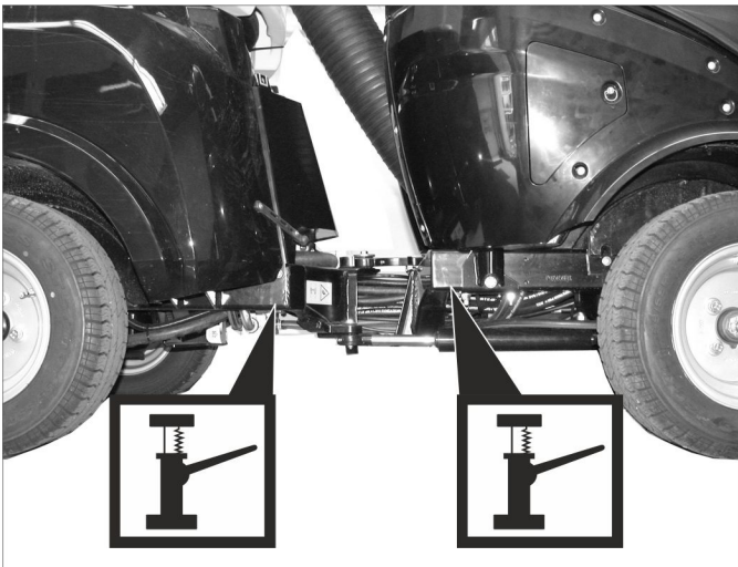
Aufnahmepunkte für Wagenheber
